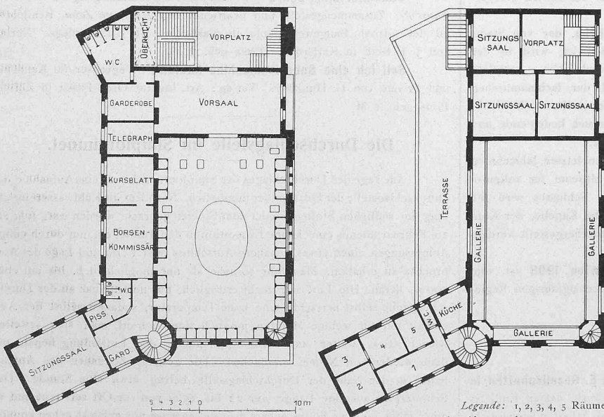
Grundrisse vom ersten und zweiten Obergeschoss. — Masstab 1 : 500.
