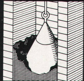
Kamin-Innenabdichtung, Patent «Schöbel-R-Verfahren».
