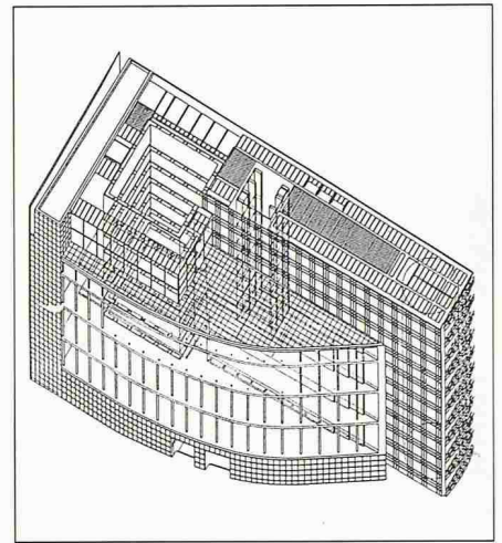
Bild 15. Axonometrische Zeichnung des Institut du Monde Arabe
