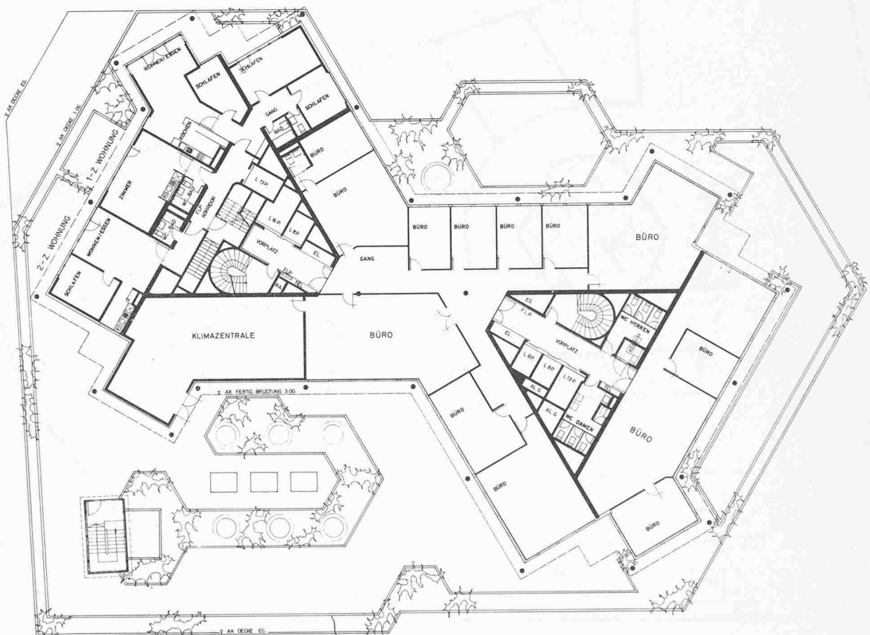
Grundriss 2. Obergeschoss 1:400
