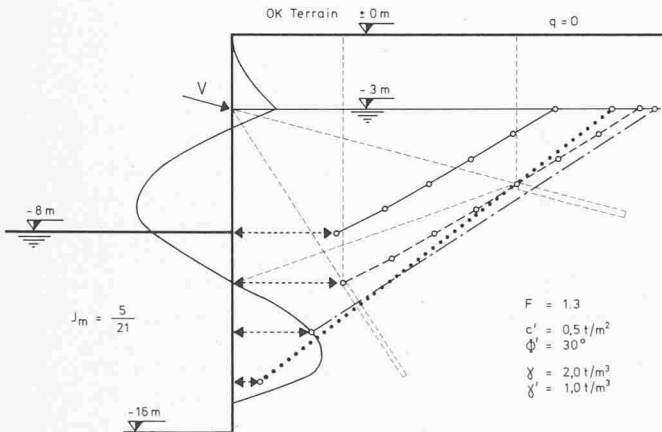
Bild 15. Beispiel zur Abschätzung der rechnerischen freien Ankerlänge l_{fr} nach der vereinfachten Formel von Janbu. Die Punkte auf den Linien sind jeweils das Ende von l_{fr} bzw. Anfang der Verankerungslänge
