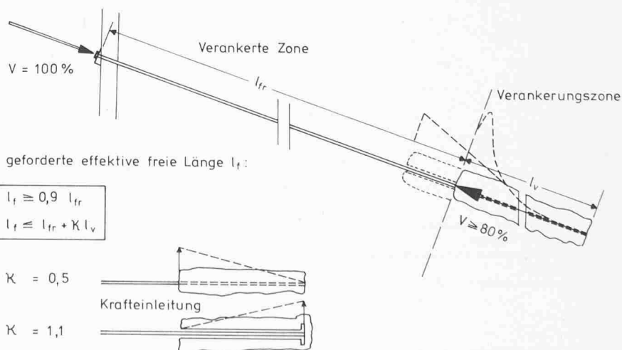
Bild 9. Schematische Darstellung der Kräfteinleitung über das Zugglied in die Verankerungszone, mit der geforderten effektiven freien Länge l_f und den Bedingungen zur Kontrolle der Grösse der eingeleiteten Kraft und deren zuverlässigen Übertragung in den Verankerungskörper
