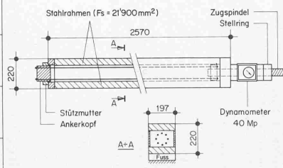
Versuchsanordnung Spannglied BBRV 8 \phi 6 , ( F_s = 221 \text{ mm}^2 , l = 2540 \text{ mm} )
