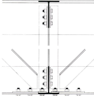
9-15 Errichtung der Dachkonstruktion. Mise on œuvre de la toiture. Erection of the roof construction.
