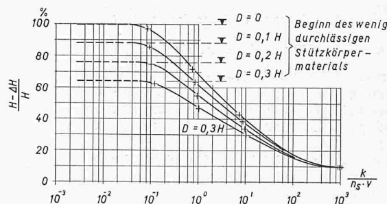
Bild 6. Darstellung des zeitlichen Verlaufes der Sickerlinie im Stützkörper während und nach einer vollständigen Absenkung des Stauspiegels (ausgehend von Vollstau). Böschungseigung des Kernes 1:0,16. Durchlässigkeitsverhältnisse: Kern und Untergrund im Verhältnis zum Stützkörper sehr klein
