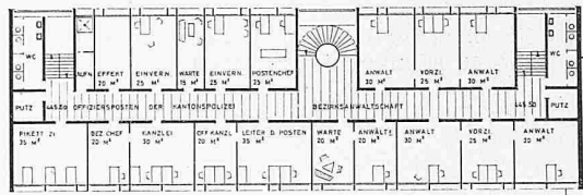
Erstes Obergeschoss
