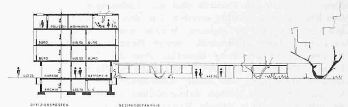
Schnitt Offiziersposten und Westfassade Gefängnis
