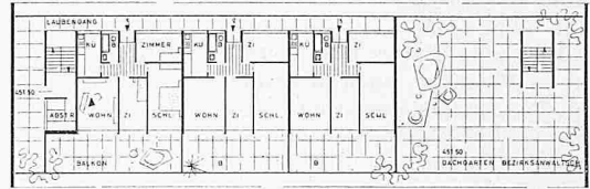
Dachgeschoss 1:700
