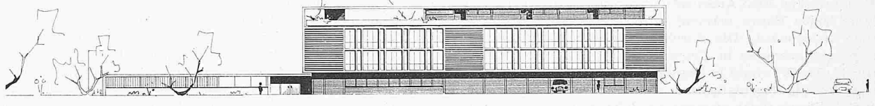
Ansicht aus Norden, Masstab 1:700
