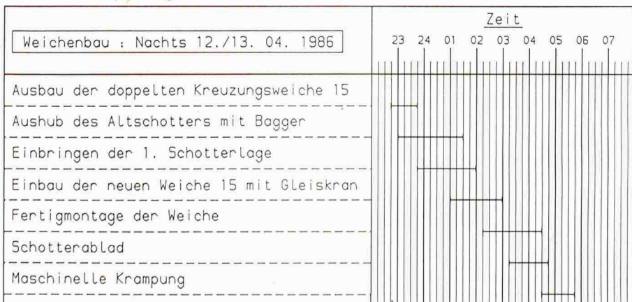
Bild 2. Ablaufplanung für den Weichenumbau
