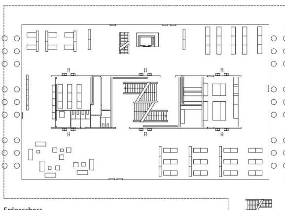
Erdgeschoss
