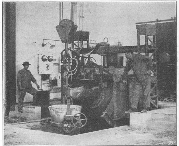
Abb. 3. Ausgussseite des Ofens, davor eine Kranflanne.
