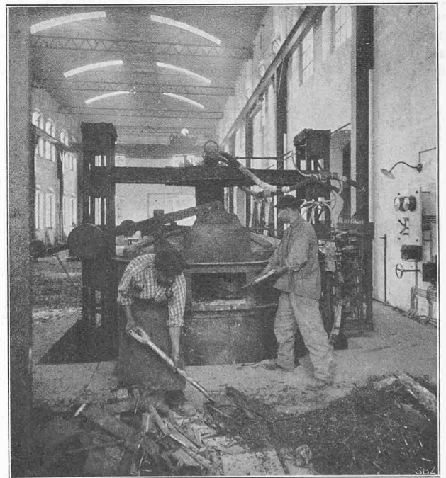
Abb. 2. Chargierseite; Einsatzmaterial.
