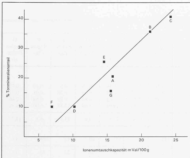
Bild 5. Zusammenhang zwischen Ionenaustauschkapazität und Tonmineralgehalt der Korngrößenfraktion <0,063 mm
