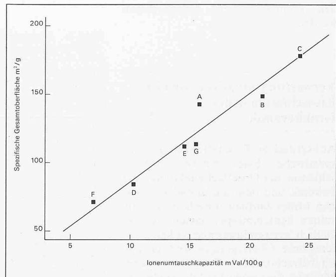
Bild 6. Zusammenhang zwischen Ionenaustauschkapazität und spezifischer Gesamtoberfläche der Korngrößenfraktion <0,063 mm
