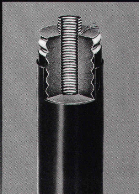
FLEXWELL- Fernwärmeleitungen
