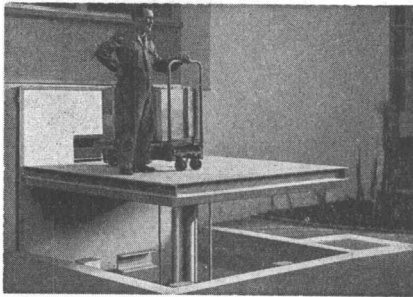
Hydraulische Hebebühne für den Warenumschlag in einem Industriebetrieb. - Hubkraft 3000 kg, Bühnengrösse 2,5 x 2,5 m.
