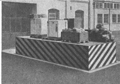
Hydraulische Hebebühne für rationelles Beladen von Fahrzeugen mit versch. Brückenhöhen. Hubkraft 6000 kg, Bühnengrösse 2,5 x 6 m.
