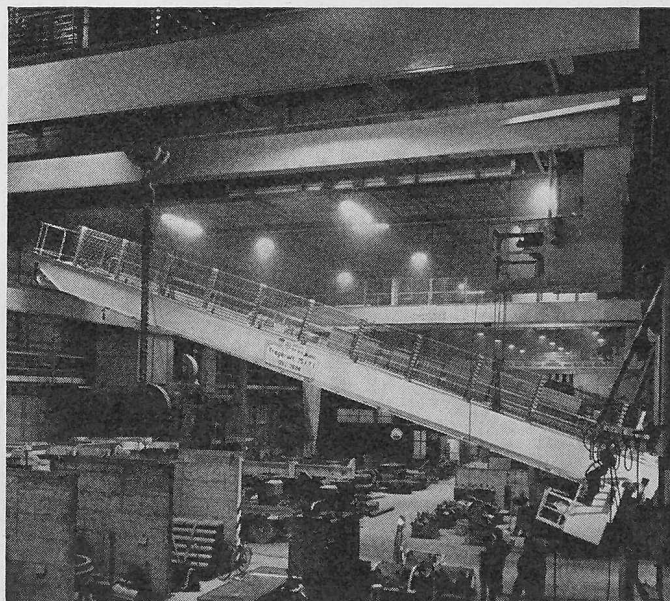
Bild 28. Aufziehen eines 25 t-Kranes. Brückenhälfte mit Stromschienen und Kabine an zwei vorbereiteten Punkten gefasst
