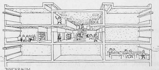
Perspektivischer Schnitt durch den Klassentrakt
