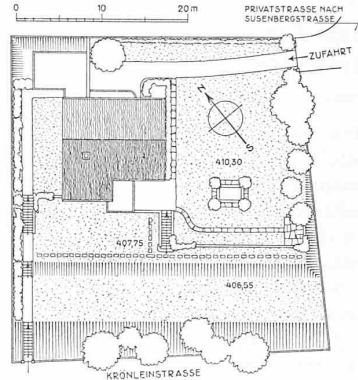
Abb. 1. Lageplan 1:800.
