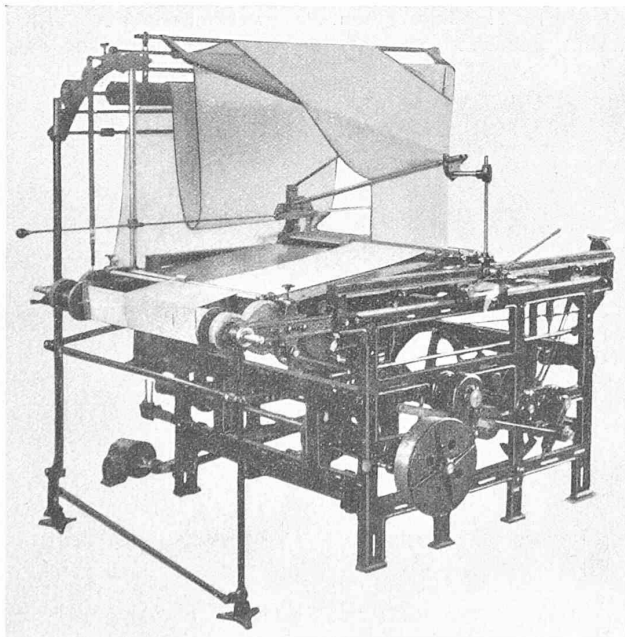
Abb. 23. Doublier-, Mess- und Legemaschine, kombiniert mit Wickelvorrichtung.
