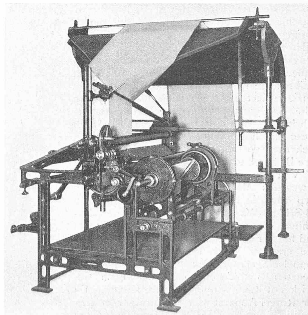
Abb. 22. Doublier-, Mess- und Wickelmaschine der Maschinenfabrik Rapperswil A.-G.
