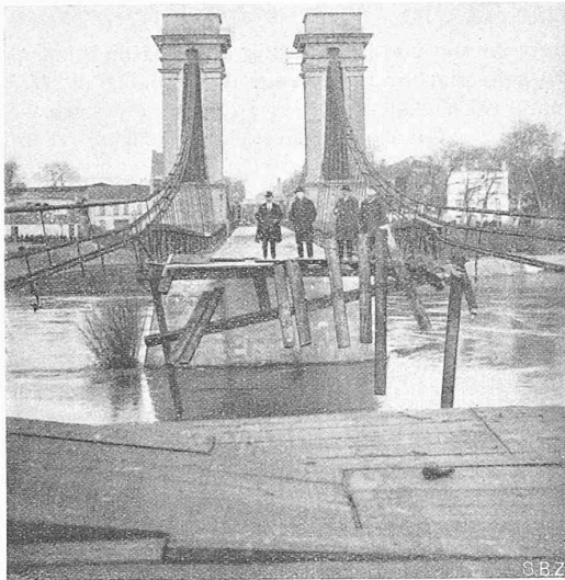
Durchbruch der Fahrbahn an der Hängebrücke über die Garonne bei Marmande in Südwest-Frankreich.
