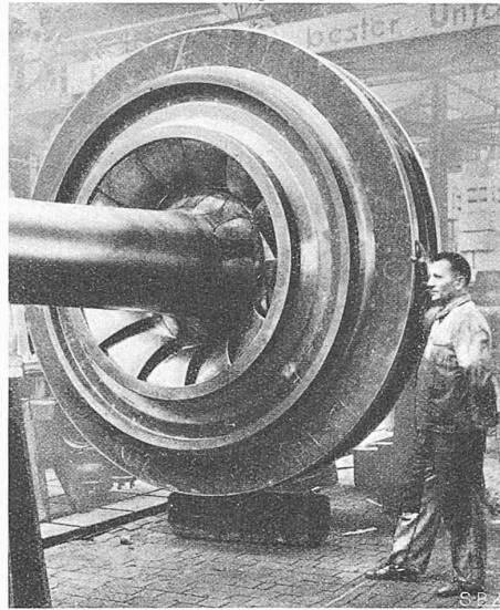
Abb. 3. Laufrad einer Pumpe für Q = 12000 l/sec bei H = 150 m für das Speicherkraftwerk Niederwartha.
