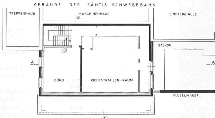
Bild 2. Geschoss 4, Grundriss 1:300
