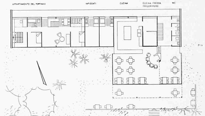
Gemeinschaftshaus Erdgeschoss, 1: 400
