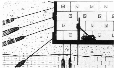
Fels- und Alluvial-Vorspanner für Hang-, Fels- und Baugrubensicherung mehrfach korrosionsgeschützte Permanentanker Auftriebsanker, Tunnelverankerungen.
