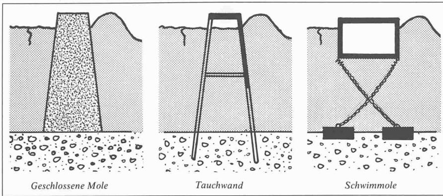
Bild 1. Drei für Hafengebauten in der Schweiz oft verwendete Molentypen
