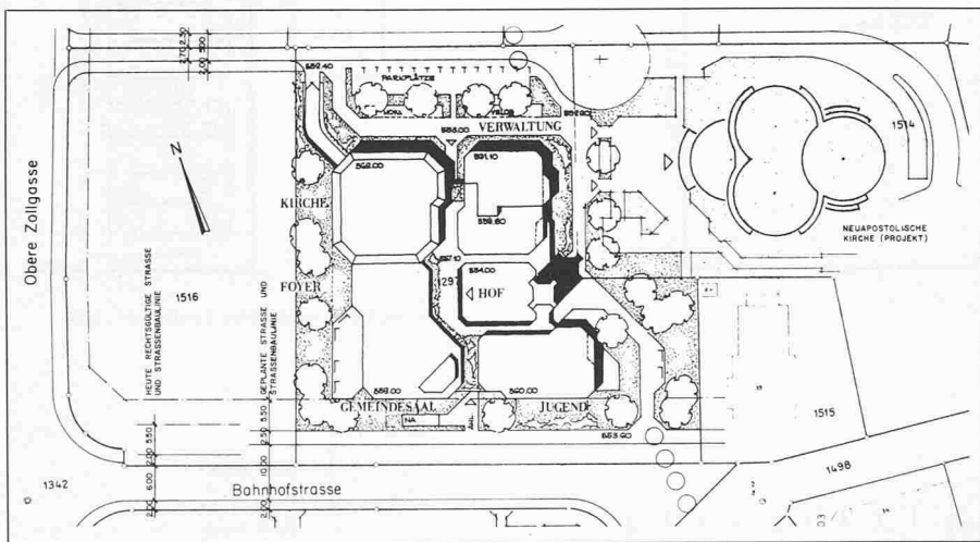
Lageplan 1:1500
