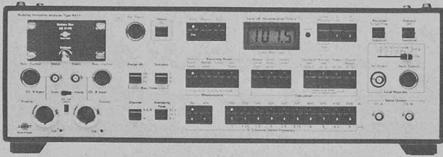
L'analyseur séquentiel Brüel & Kjaer type 4417.
