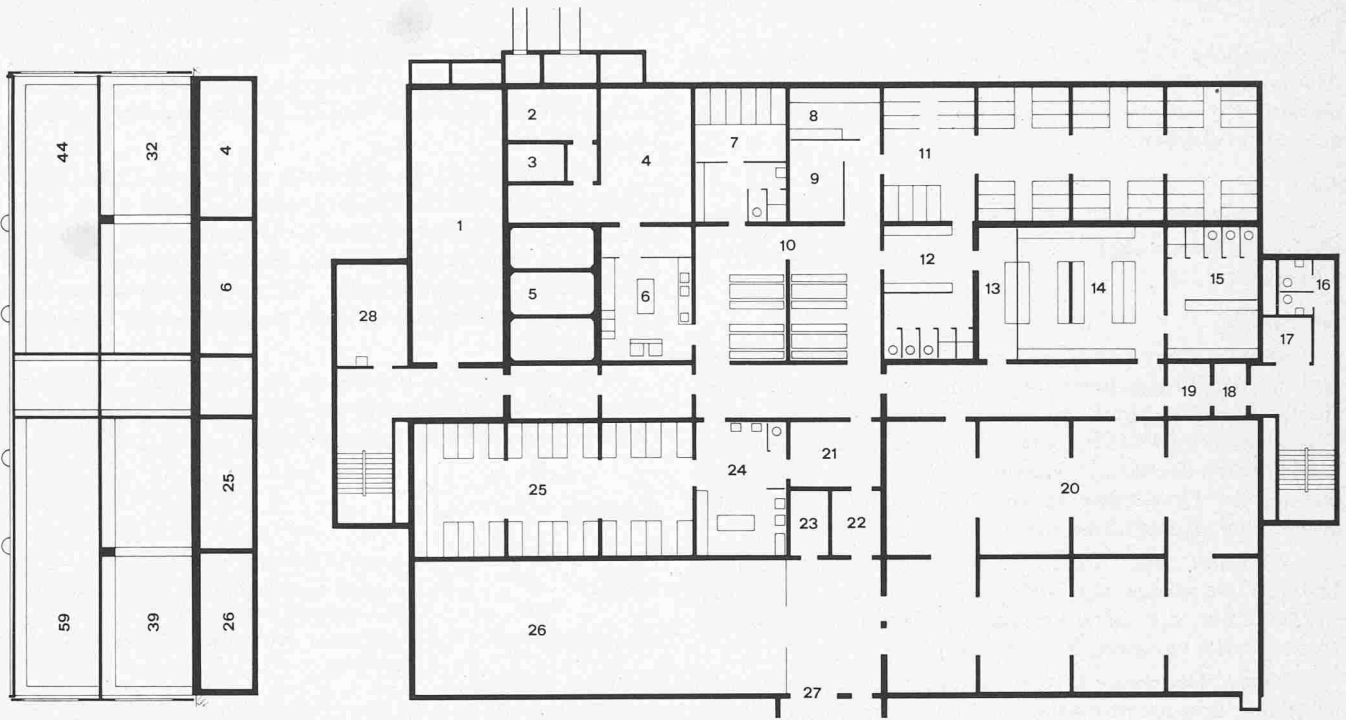
Werkstatt, Schnitt Untergeschoss 1:400. 1 Verteilraum, Lüftung, Heizung, 2 Notstrom, 3 Tank, 4 Lüftung, 5 Wassertank, 6 Küche, 7 Schlafrum Frauen, 8 Büro, 9 Büro, 10 Aufenthaltsraum, 11 Schlafrum Männer, 12 Waschraum, 13 Garderobe Frauen, 14 Garderobe Männer, 15 Waschraum, 16 WC, 17 Putzraum, 18 Schleuse, 19 Reinigung, 20 Schutzraum, Velo-/Mopedraum, 21 Reinigung, 22 Schleuse, 23 Materialraum, 24 Behandlung, 25 Sanitätsposten, 26 Geräteraum, 27 Rampe 28 Putzraum, Reserve
