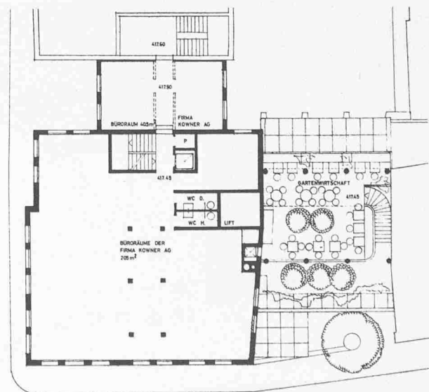
2. Obergeschoss 1:370
