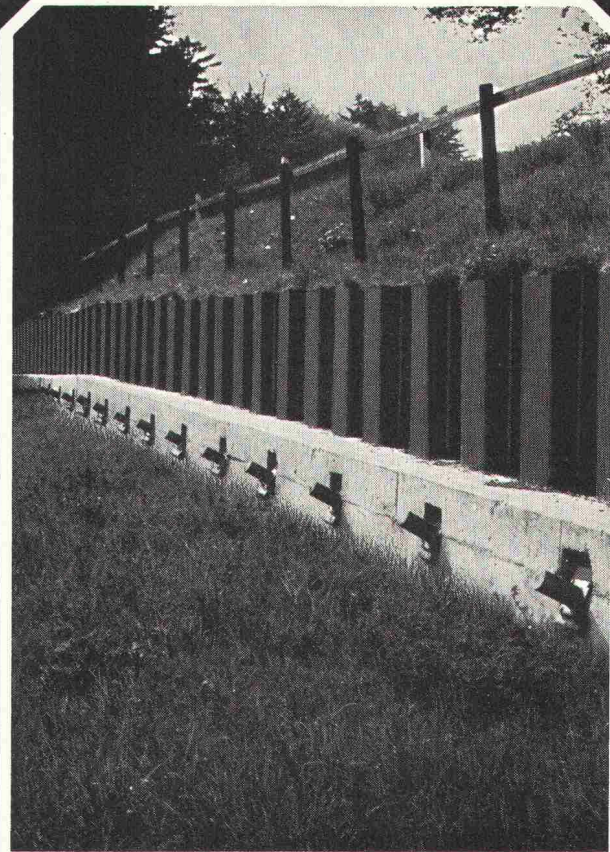
Rutschsanierung Hüntwangen
