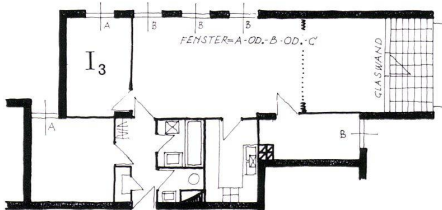
Standardwohnung, Typ I3 Variationsmöglichkeiten bezüglich Trennwände, Fenster, Installationen
