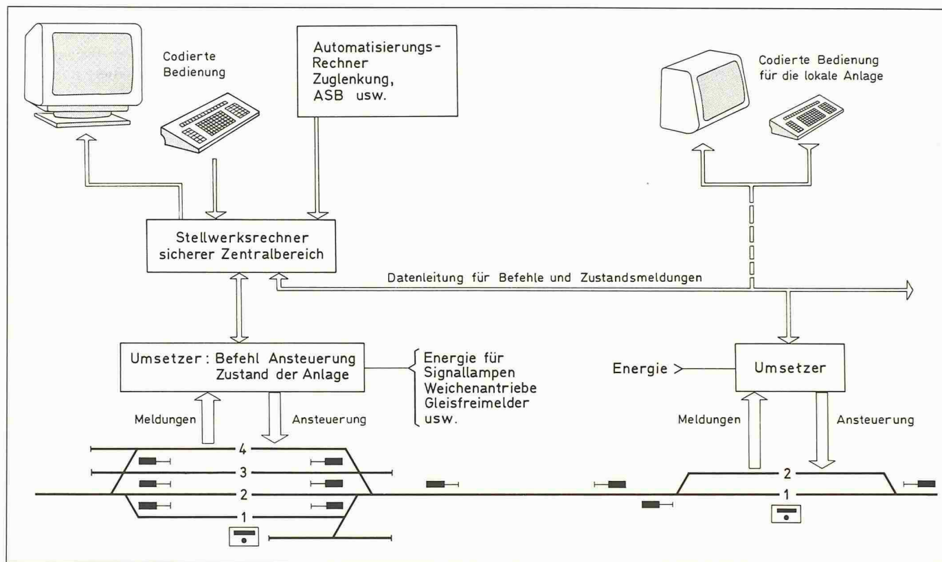
Bild 1. Elektronisches Stellwerk 2000
