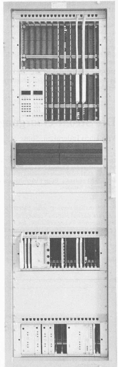
Bild 5. Fernwirkzentrale TELEGYR®709S
