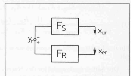
Bild 2. Aufgeschnittener Regelkreis
