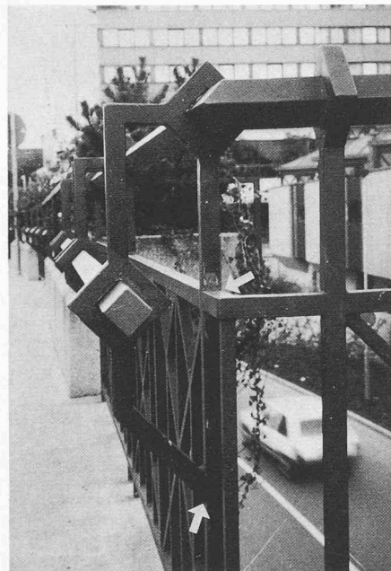
Bild 13. Elemente aus Gusseisen mit Kugelgraphit an einem Geländer beim Bahnhof Lörrach. Die von Vierkantrohren durchdrungenen Gusselemente sind mit den Pfosten verschweisst. (Werkfoto Giesserei Trikes, Lörrach)
