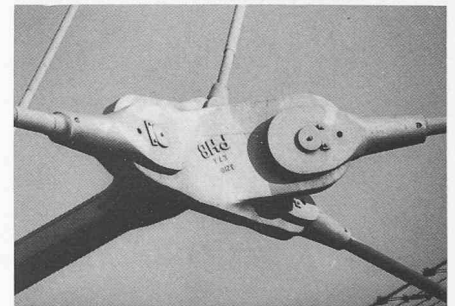
Bild 9. Verteilerknoten aus Stahlguss in der Seilnetzkonstruktion des Olympiadaches in München (Werkfoto PHB-Weserhütte, St. Ingbert)
