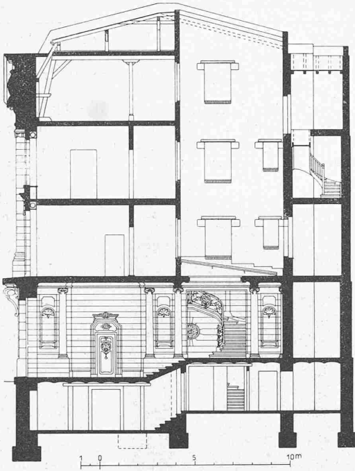
Abb. 4. Schnitt durch den Haupttrakt an der Freiengasse. Masstab 1:250.
