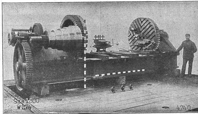
Radsatz-Drehbank.
