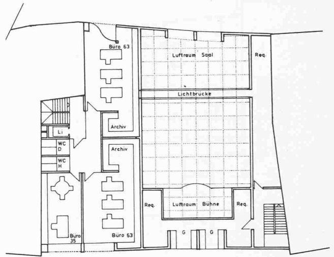
Grundriss 2. Obergeschoss 1:400
