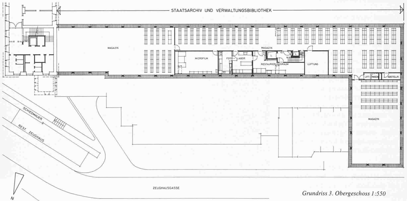
Grundriss 2. Obergeschoss 1:550
