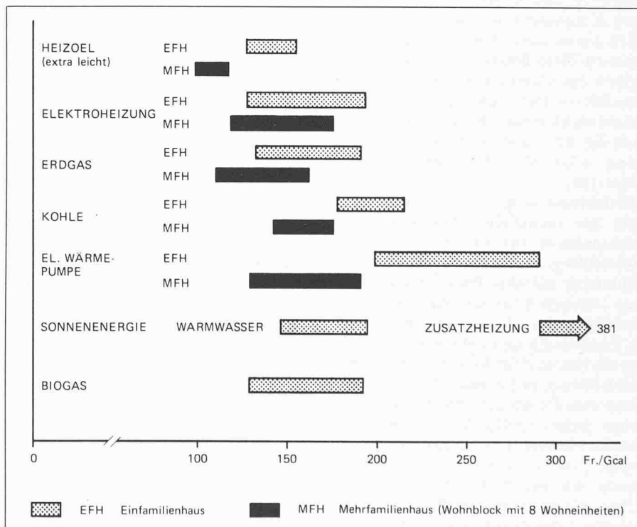
Bild 3. Wärmegestellungskosten verschiedener Heizsysteme (Stufe Nutzenergie) bei Einzelgebäudeheizung (Preisbasis 1977)
