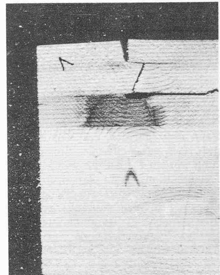
Bild 13. Lokale Fäulnis im Innern des Messbalkens, im Verlaufe eines Jahres verursacht durch Lenzites-Befall nach Durchfeuchtung im Bereich eines Risses auf der Oberseite
