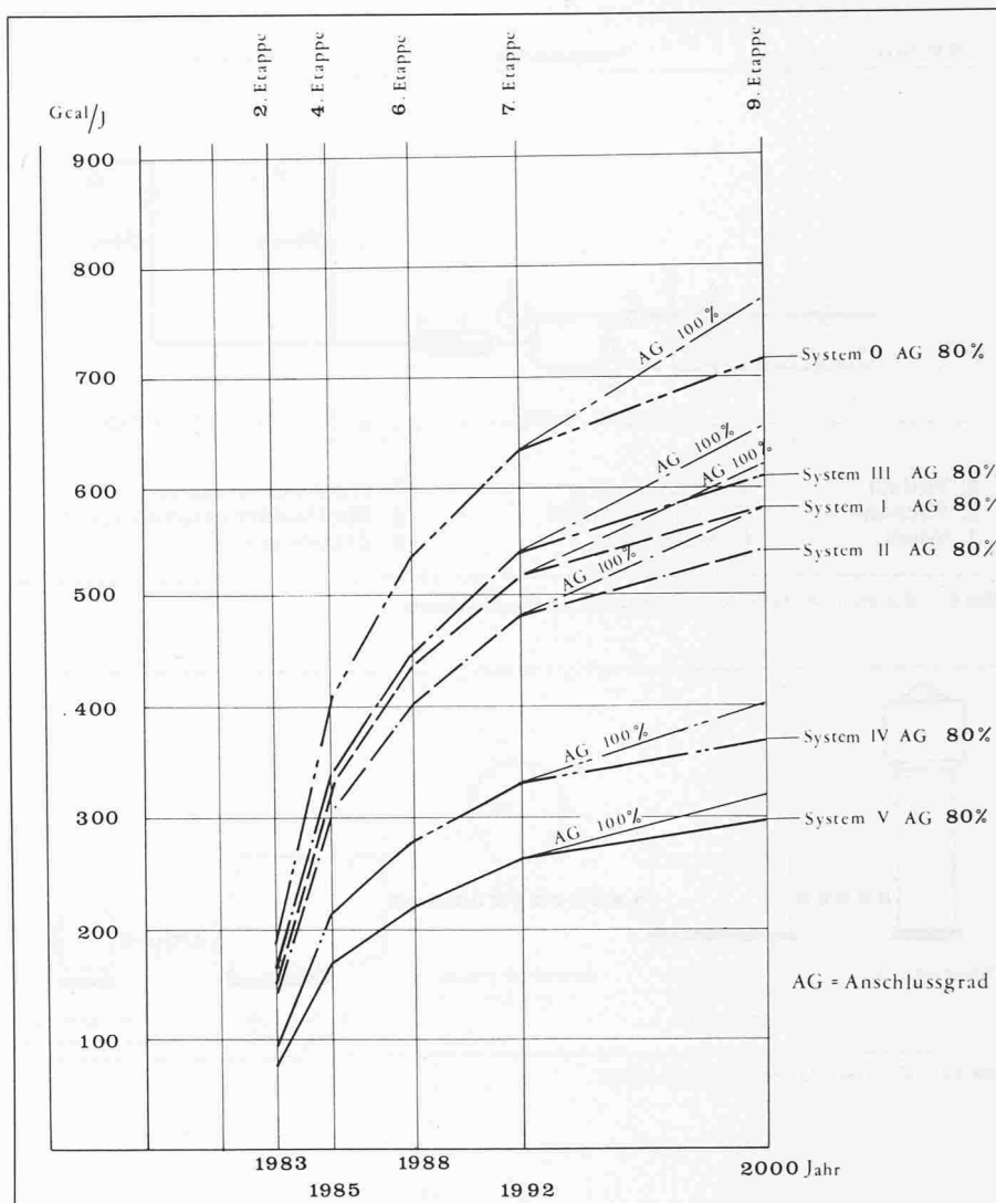
Bild 7. Netzverluste
