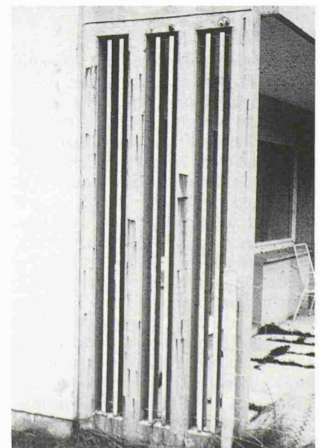
Bild 2. Stützenquerschnitte 12 \times 12 cm, Baujahr 1964.
