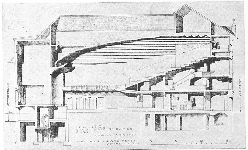
Abb. 14. Längsschnitt des Capitol-Theaters in Bern. — Masstab 1 : 400.
