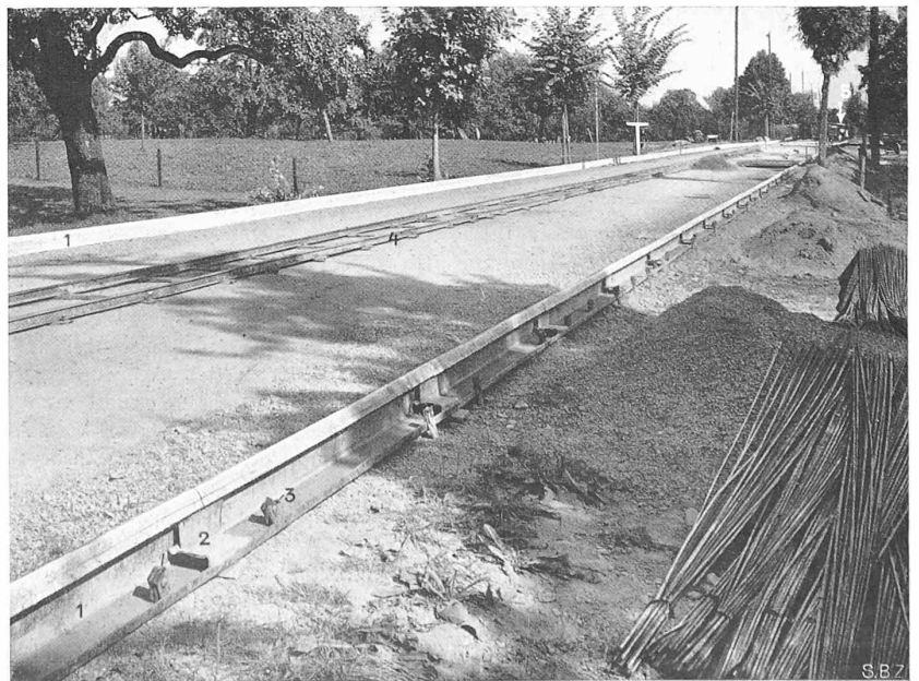
Abb. 7. Laufschielen des Strassenfertigers von Jos. Voegele ((Mannheim). 1 Schiene, 2 Stoss mit Keil und Keilplatte versteift, 3 „Heringe“ zur Verankerung in Boden, 4 Transportgeleise, 5 Einbaustelle.
