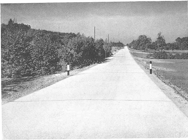
Abb. 11. Betonstrasse Arbon-Amriswil.
