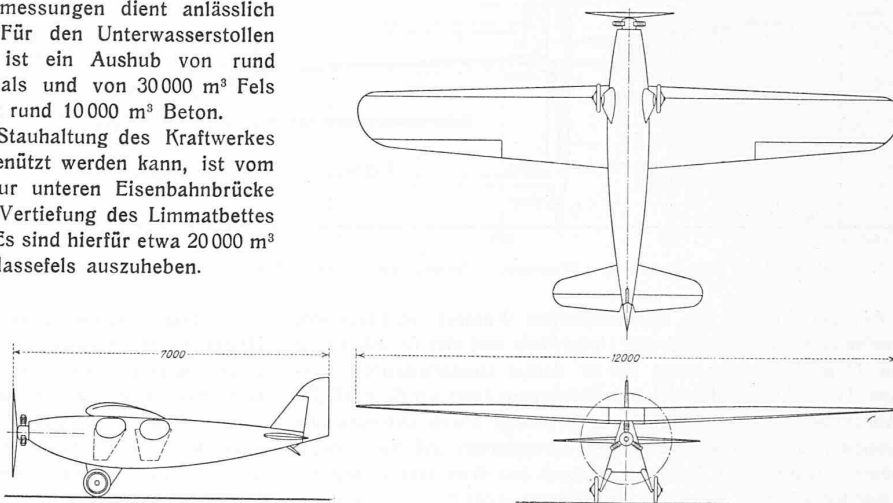
Abb. 1 und 2. Ansicht und Masskizze 1:150 des Sportflugzeugs „Korsa I“.
