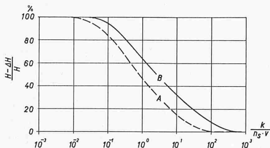
Bild 3. Allgemeine Darstellung der Lage der Sickerlinie (z. B. beim Kern) z. Zeit T in Abhängigkeit von k/n_s \cdot v
