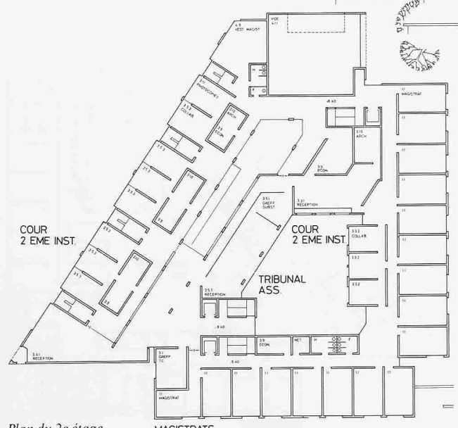
Plan du 2e étage
