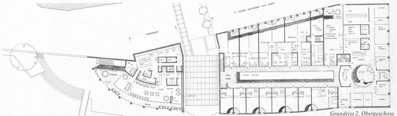
Grundriss 2. Obergeschoss
