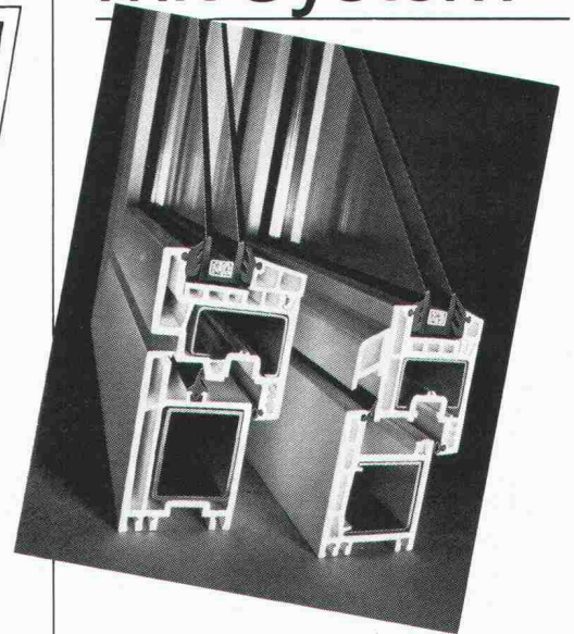
2flügliges Dreh-/Kipfenster ohne Setzstück
